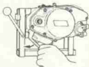
FIG. 11 Rimozione seeger pignone catena Chain sprocket snap ring removal
