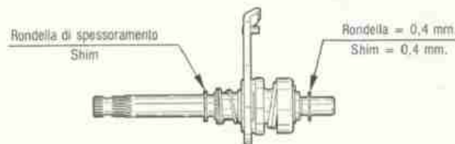
FIG. 29 Gruppo selettore Gear-box selector
