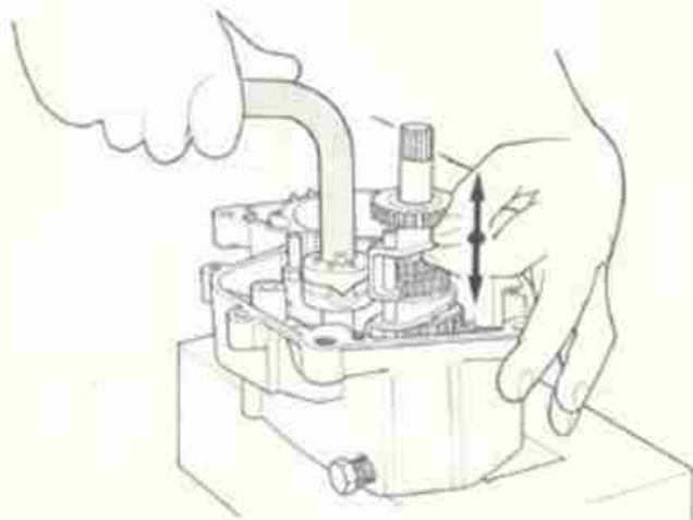
FIG. 38 Controllo cambio Gear-box check
