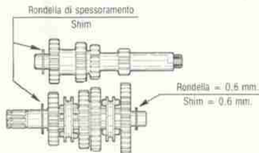
FIG. 27 Cambio a 4 velocità 4 speed gear-box
