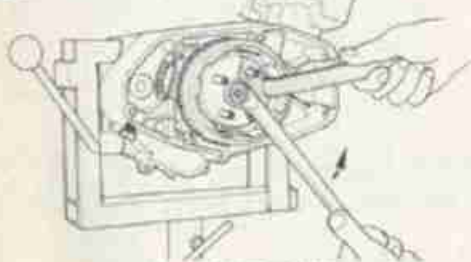
FIG. 14 Rimozione dado Nut removal
