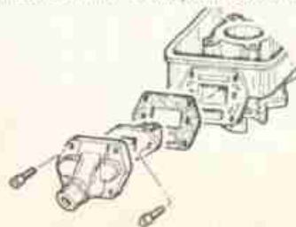
FIG. 52 Gruppo lamelle Reed valve assy
