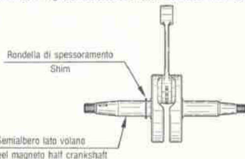
FIG. 25 Imbiellaggio Crankshaft
