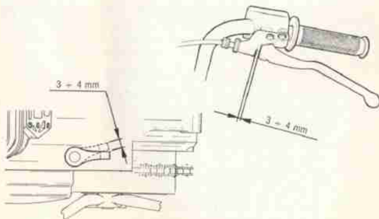
FIG. 4 Controllo gioco frizione Clutch clearance check
