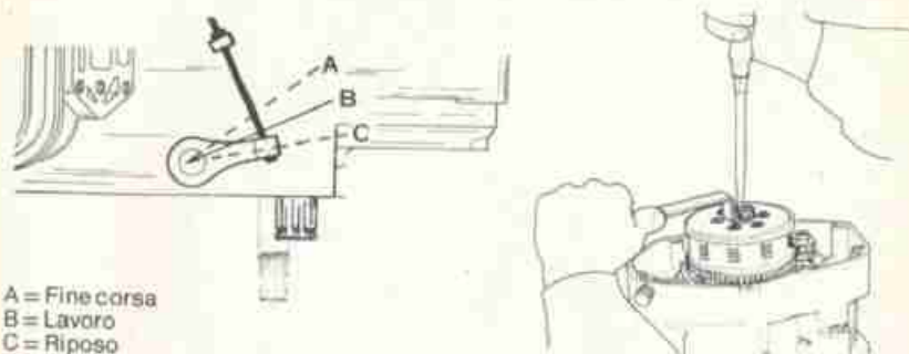
FIG. 46 Registrazione frizione Clutch adjustment
